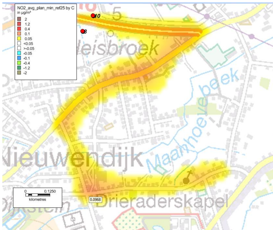
Figuur 5-41 detail wegen met aantoonbare jaargemiddelde impact NO2 (worst case berekend op basis van emissiefactoren 2025)
