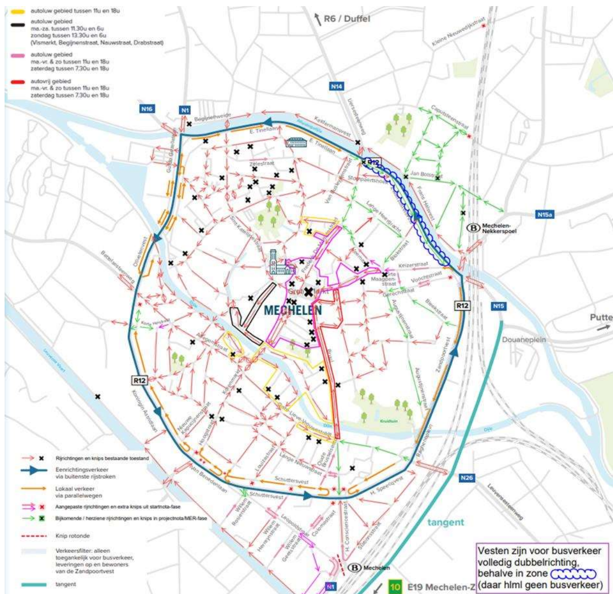
Figuur 2: Circulatiemaatregelen i.h.k.v. Herinrichting Mechelse Vesten – scenario 4
