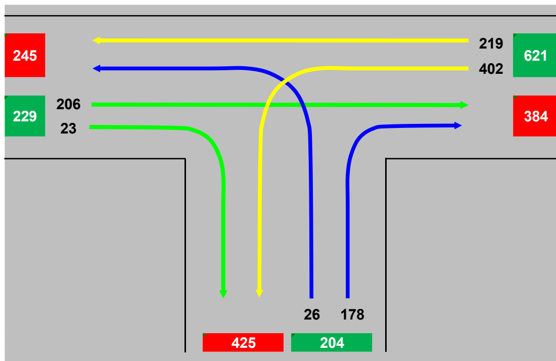
Figuur 5-20 Intensiteiten Mechelsesteenweg X Meidoornstraat, toekomstige toestand, avondspits (16:30-17:30)
