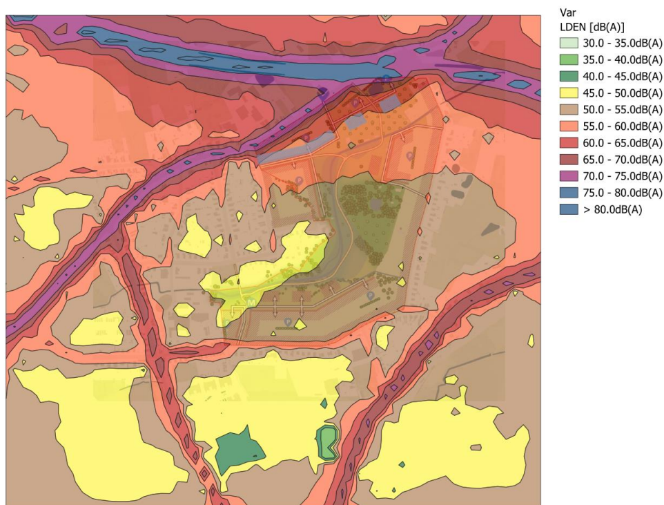
Figuur 5-35 Maenhoevevelden: Lden geluidscontourkaart (geplande toestand)
