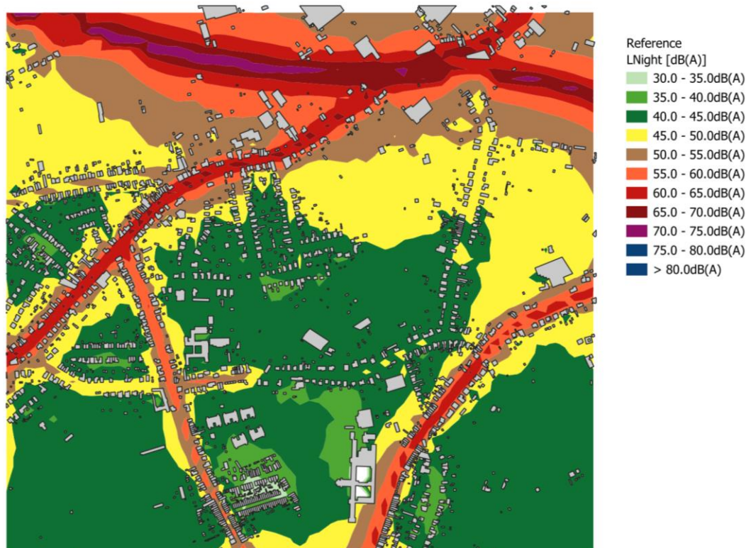
Figuur 5-31 Geluidscontourenkaart Referentiesituatie wegverkeer Lnight
