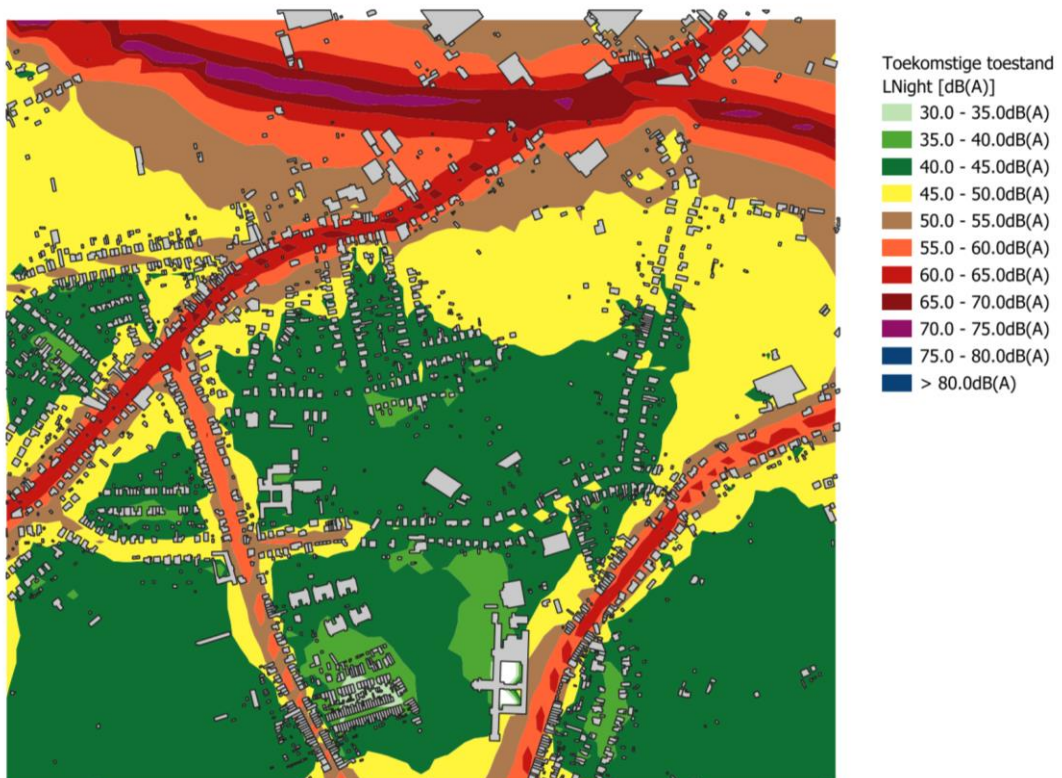
Figuur 5-33 Geluidscontourenkaart Geplande situatie wegverkeer Lnight
