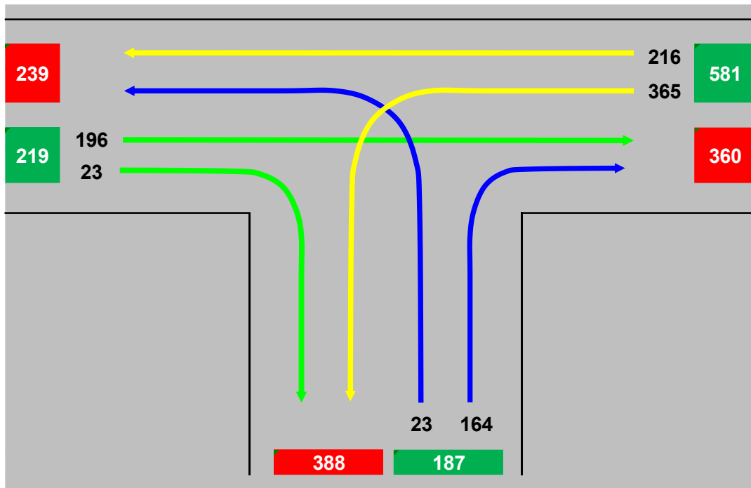
Figuur 5-15 Intensiteiten Mechelsesteenweg X Meidoornstraat, referentie, avondspits (16:30-17:30)
