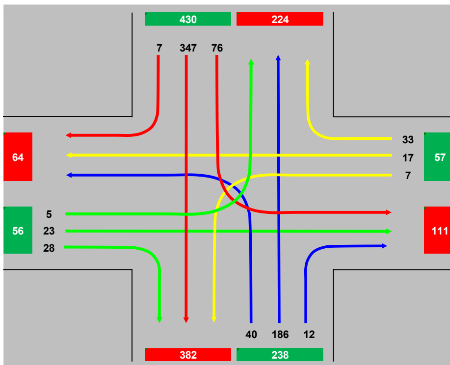
Figuur 5-22 Intensiteiten Berkelei X Meidoornstraat, referentie, avondspits (16:30-17:30)
