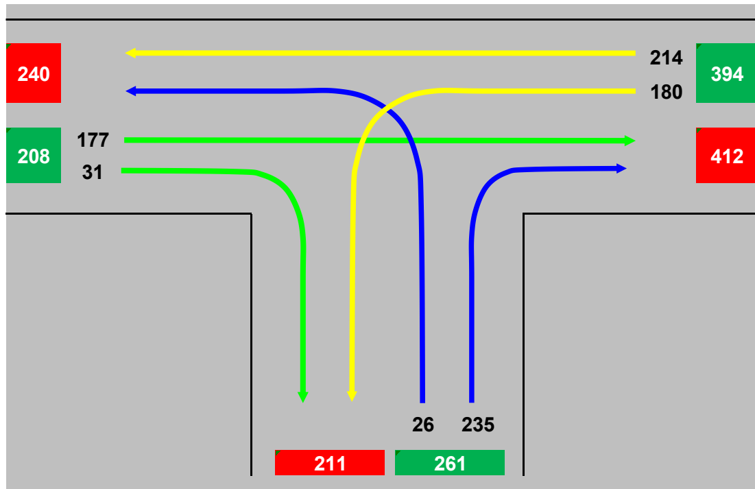
Figuur 5-14 Intensiteiten Mechelsesteenweg X Meidoornstraat, referentie, ochtendspits (08:00-09:00)
