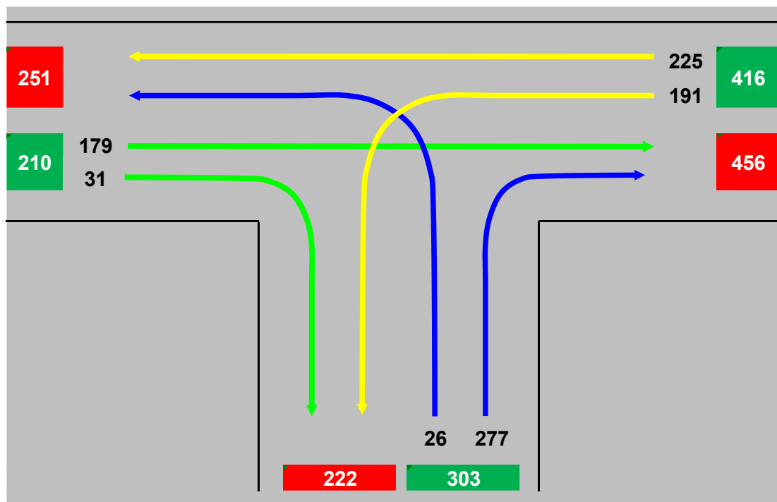
Figuur 5-19 Intensiteiten Mechelsesteenweg X Meidoornstraat, toekomstige toestand, ochtendspits (08:00-09:00)
