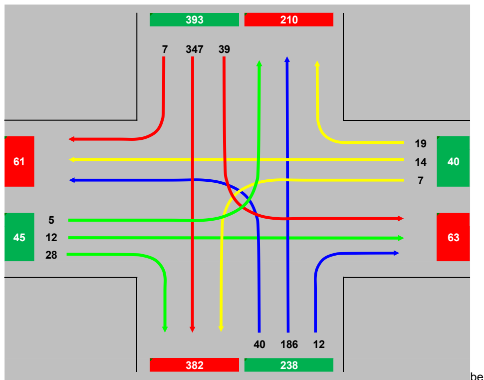
Figuur 5-17 Intensiteiten Berkelei X Meidoornstraat, referentie, avondspits (16:30-17:30)
