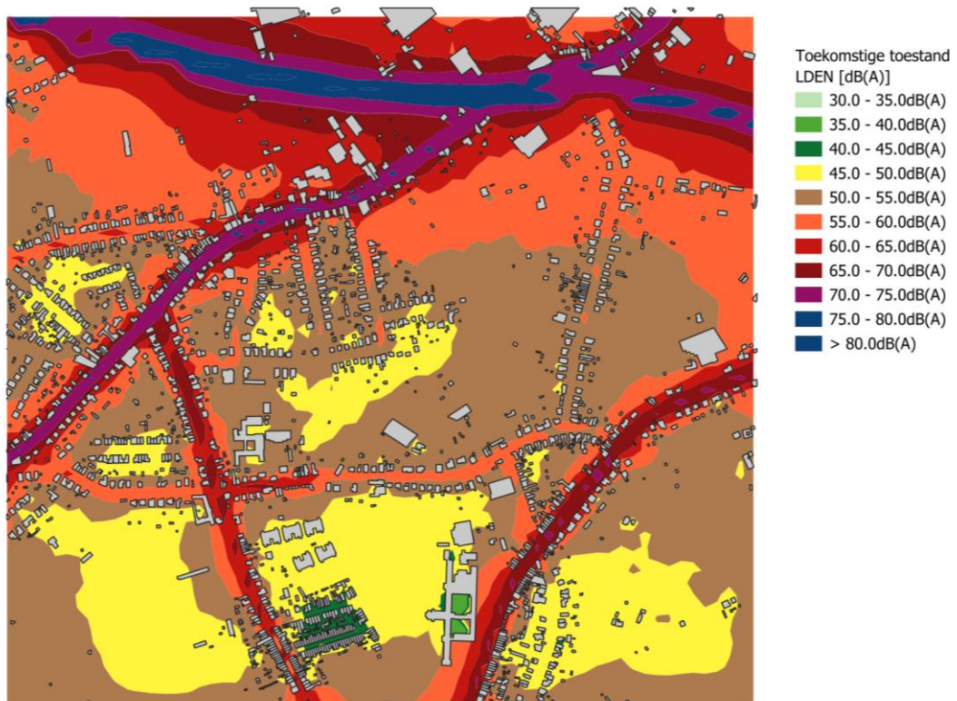
Figuur 5-32 Geluidscontourenkaart Geplande situatie wegverkeer Lden
