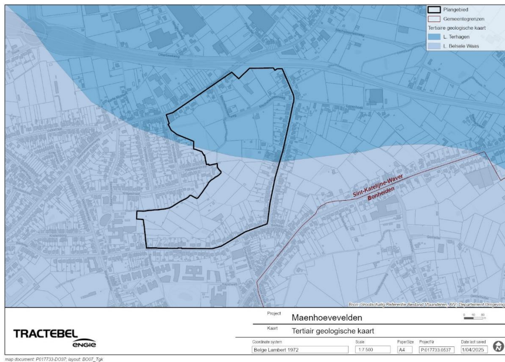
Figuur 5-42 Maenhoevevelden gesitueerd op de Tertiair geologische kaart
