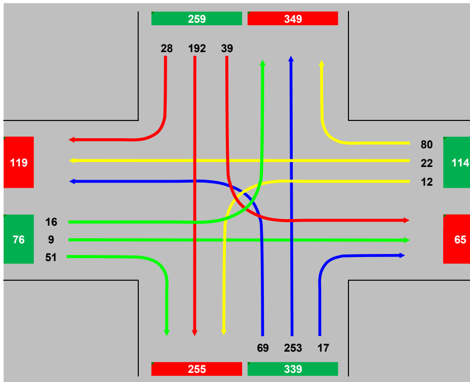
Figuur 5-21 Intensiteiten Berkelei X Meidoornstraat, referentie, ochtendspits (08:00-09:00)
