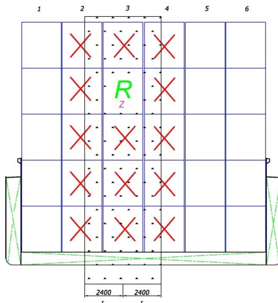
Vooraanzicht
