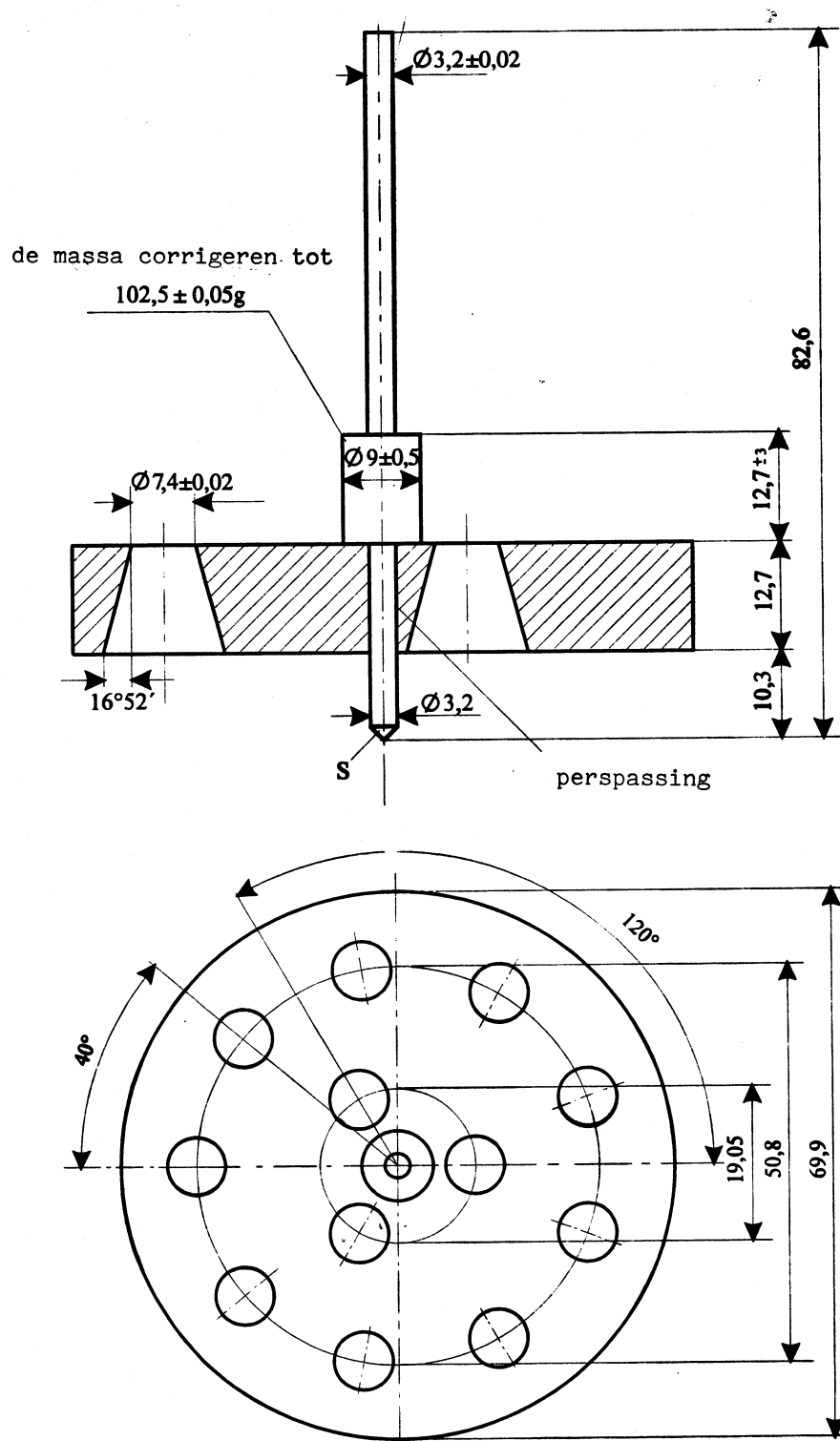
Figuur 1 Penetrometer
