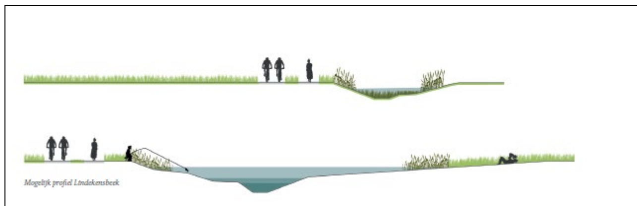
Figuur 20. Lindekensbeek: voorgestelde ontwikkeling (Open Ruimte Perspectief Nijlen, 2018)
