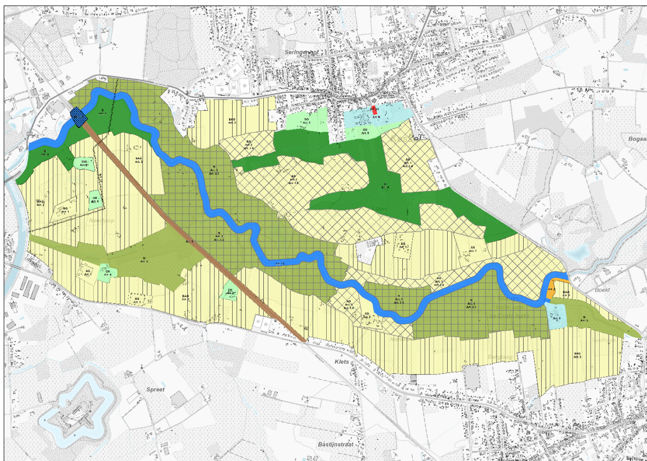
Figuur 6-2 Overzicht ontwerpplan
